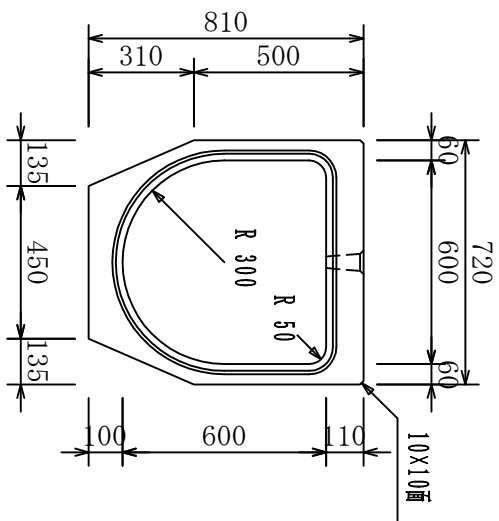
正面图
