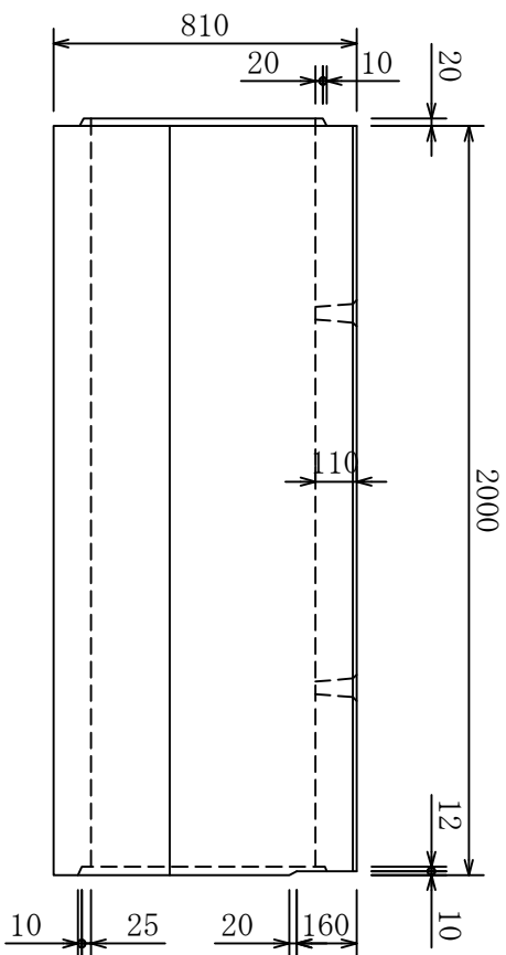
侧面图
