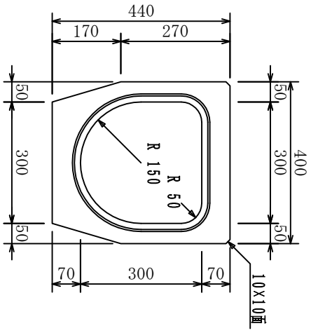
正面图
